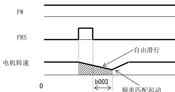
(例2) 频率匹配起动
