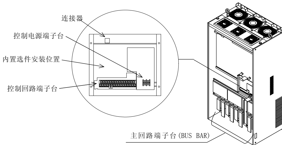
取下表面盖板·端子台盖板后的状态
