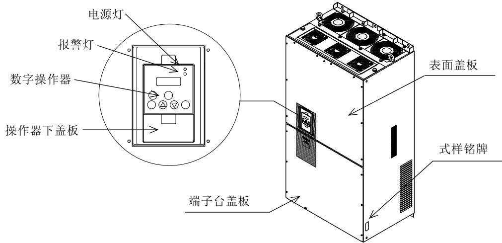
出厂时的外观
