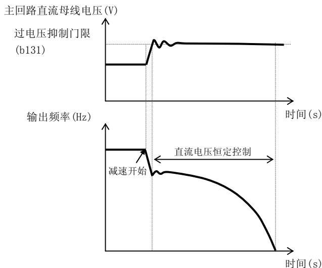
例 1) 设定 b130=01 时
